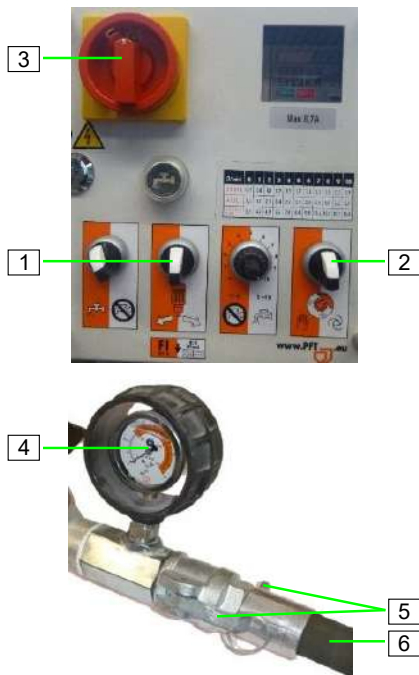
Abb. 78: Mörtelschlauch abkuppeln
