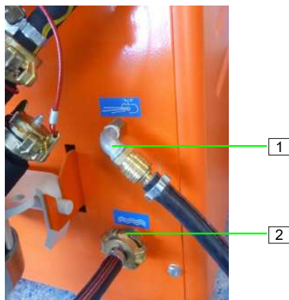
Abb. 76: Luftschlauch anschließen
