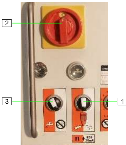
Abb. 41: Maschine einschalten
