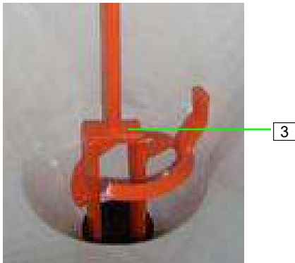
Abb. 74: Mischwendel entnehmen
