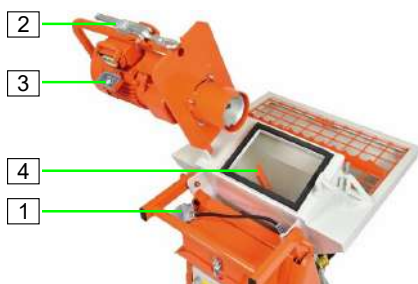
Abb. 82: Motorrippflansch öffnen
