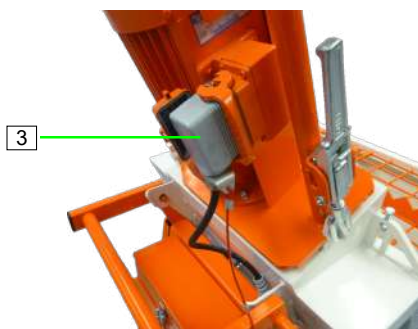
Abb. 35: Motoranschlusskabel anschließen
