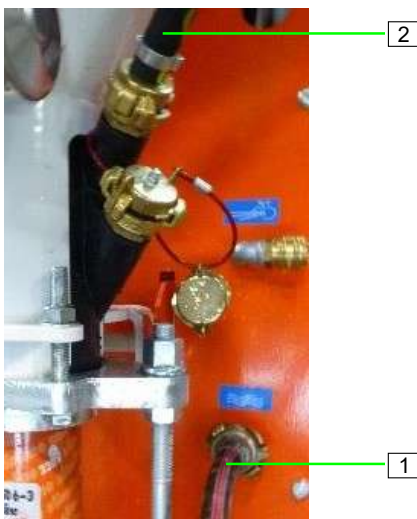
Abb. 73: Wasserzufuhr trennen
