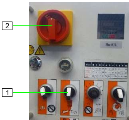
Abb. 67: Maschine ausschalten
