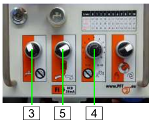
Abb. 69: Maschine einschalten
