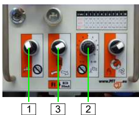
Abb. 57: Einschalten
