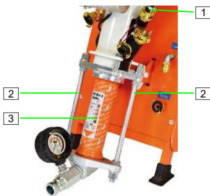
Abb. 87: Pumpeneinheit abnehmen
