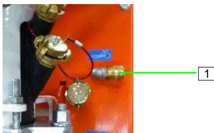
Abb. 48: Luftschlauch anschließen
