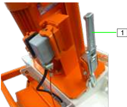
Abb. 6: Schnellverschluss schließen
