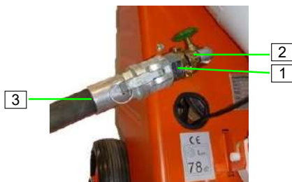
Abb. 45: Mörtelschläuche vorbereiten
