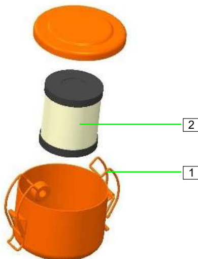
Abb. 103: Luftfilter reinigen
