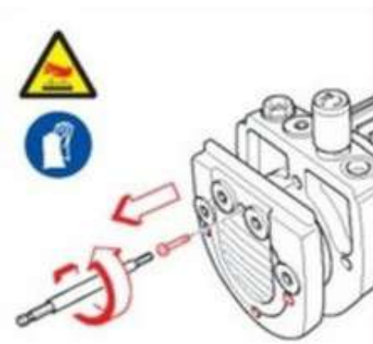
Abb. 104: Seitendeckel lösen
