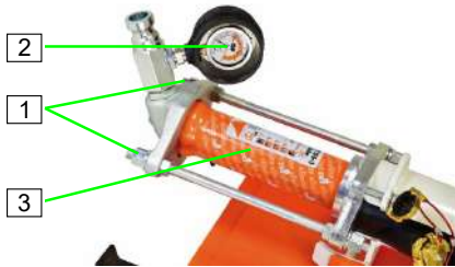
Abb. 108: Pumpeneinheit abnehmen
