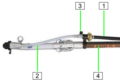
Abb. 49: Spritzgerät
