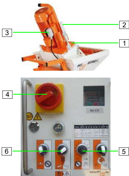
Abb. 85: Mischrohr reinigen
