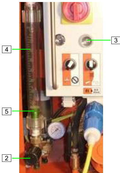
Abb. 43: Wassermenge einstellen
