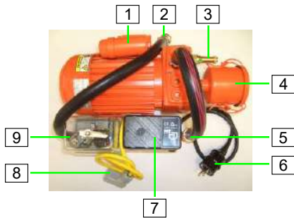
Abb. 18: Baugruppe Luftkompressor
