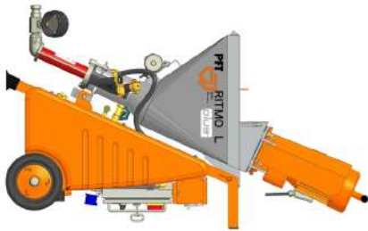
Abb. 86: Maschine umlegen
