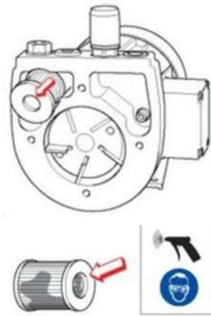
Abb. 105: Filter druchblasen
