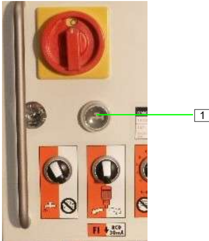
Abb. 44: Mischzone wässern
