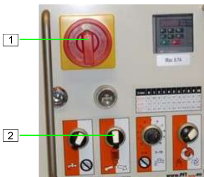
Abb. 92: Rückwärtslauf
