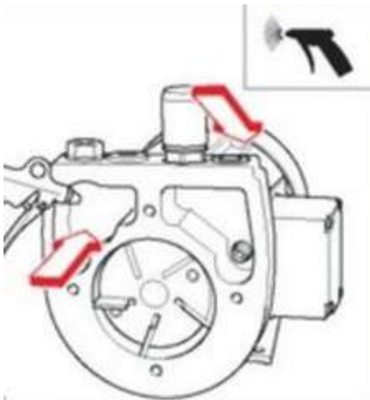
Abb. 106: Luftfiltergehäuse ausblasen
