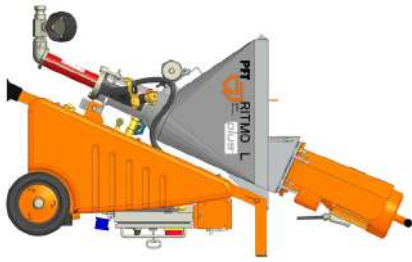
Abb. 107: Maschine umlegen
